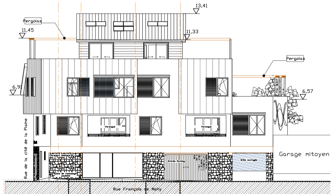
PC5 Façade Ouest 1:150
